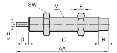
沒帶塑膠頭 No head
