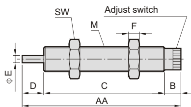
沒帶塑膠頭 No head
